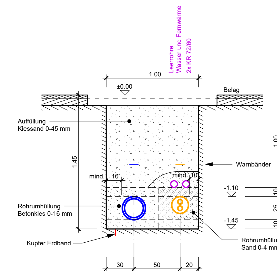
Grabenprofil 2. Bauetappe 1:25
