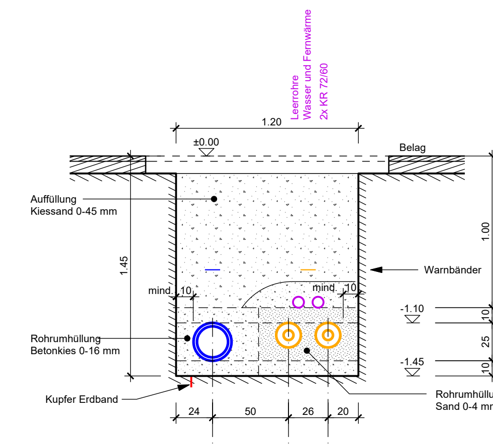
Grabenprofil 1. Bauetappe 1:25
